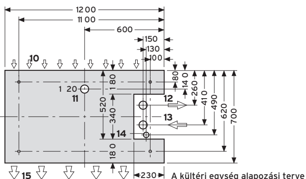
A kültéri egység alapozási terve
